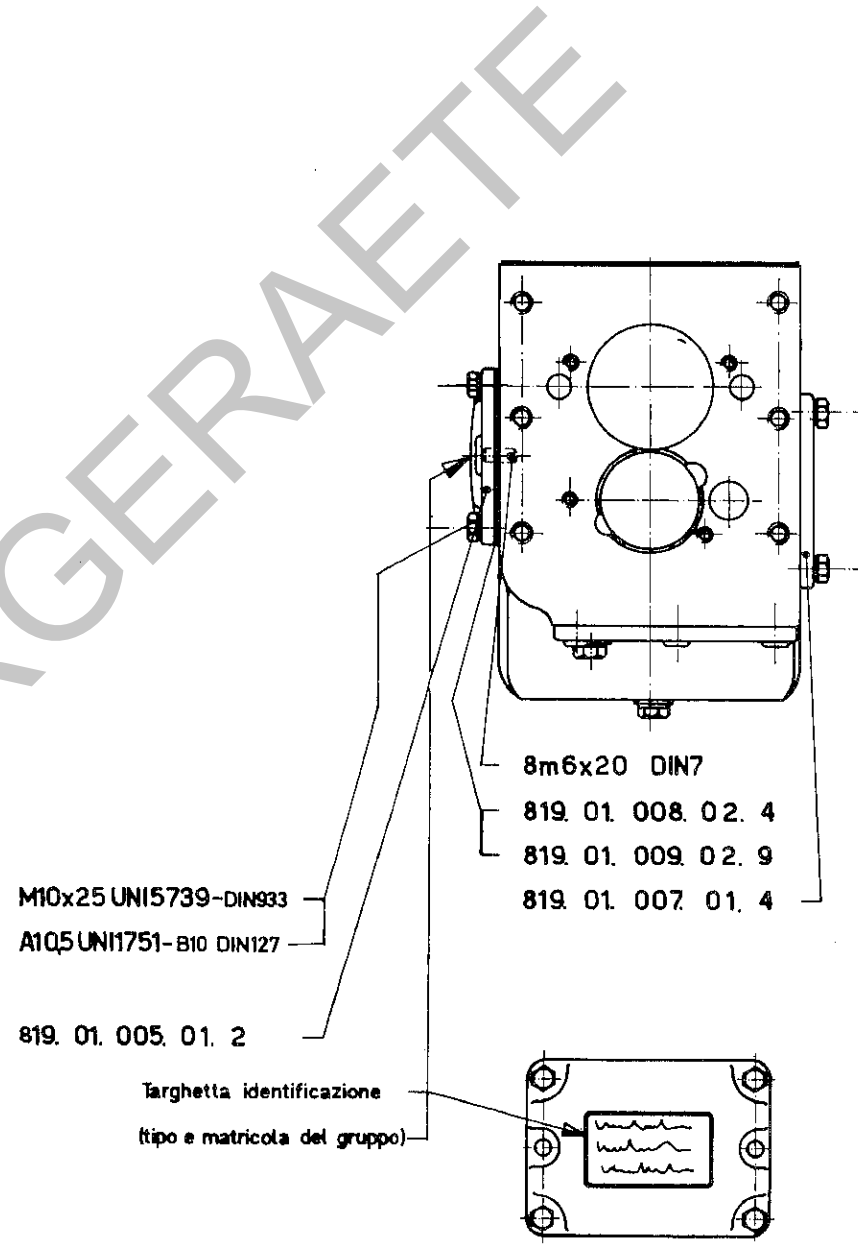
B 41 Getriebe (mit Allradantrieb) Baugruppe 01, Getriebegehäuse mit Deckel 819. 01. 000. 05. 2 Bildtafel Nr. 23
