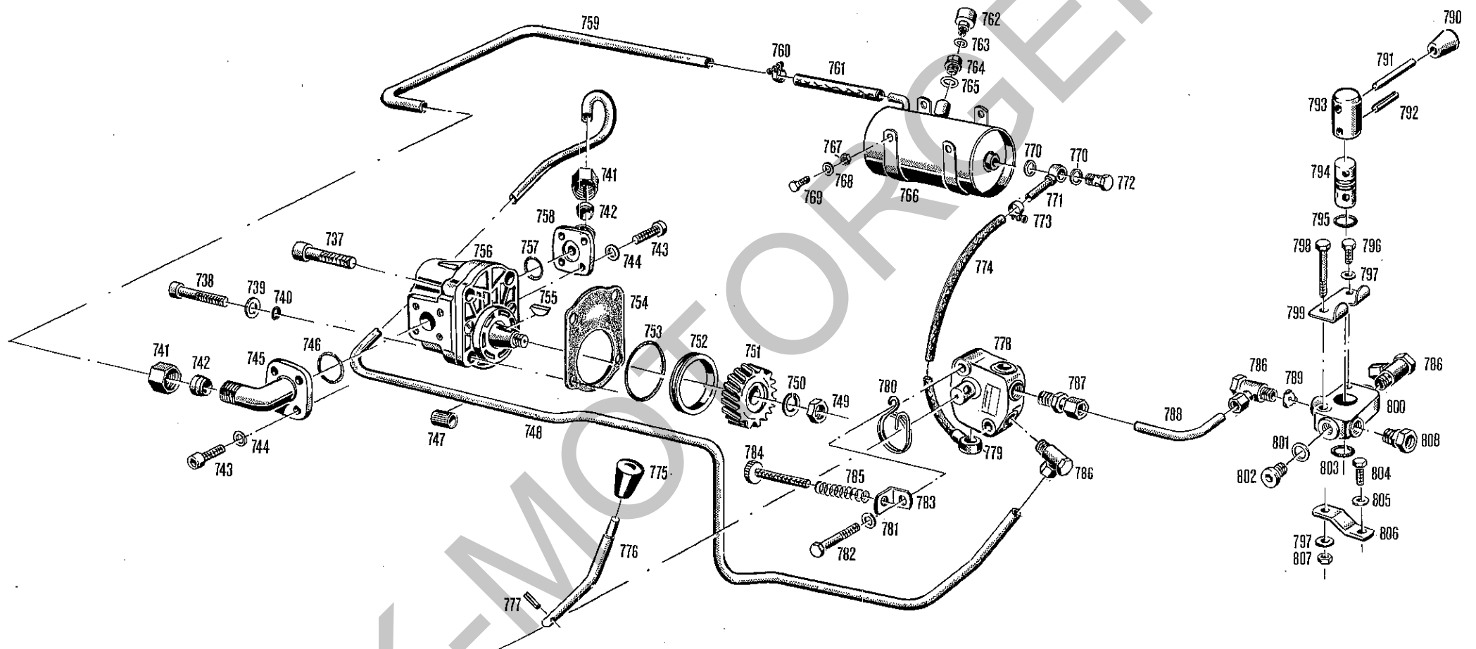
Bildtafel No. 11 Bis B 18-1222325
