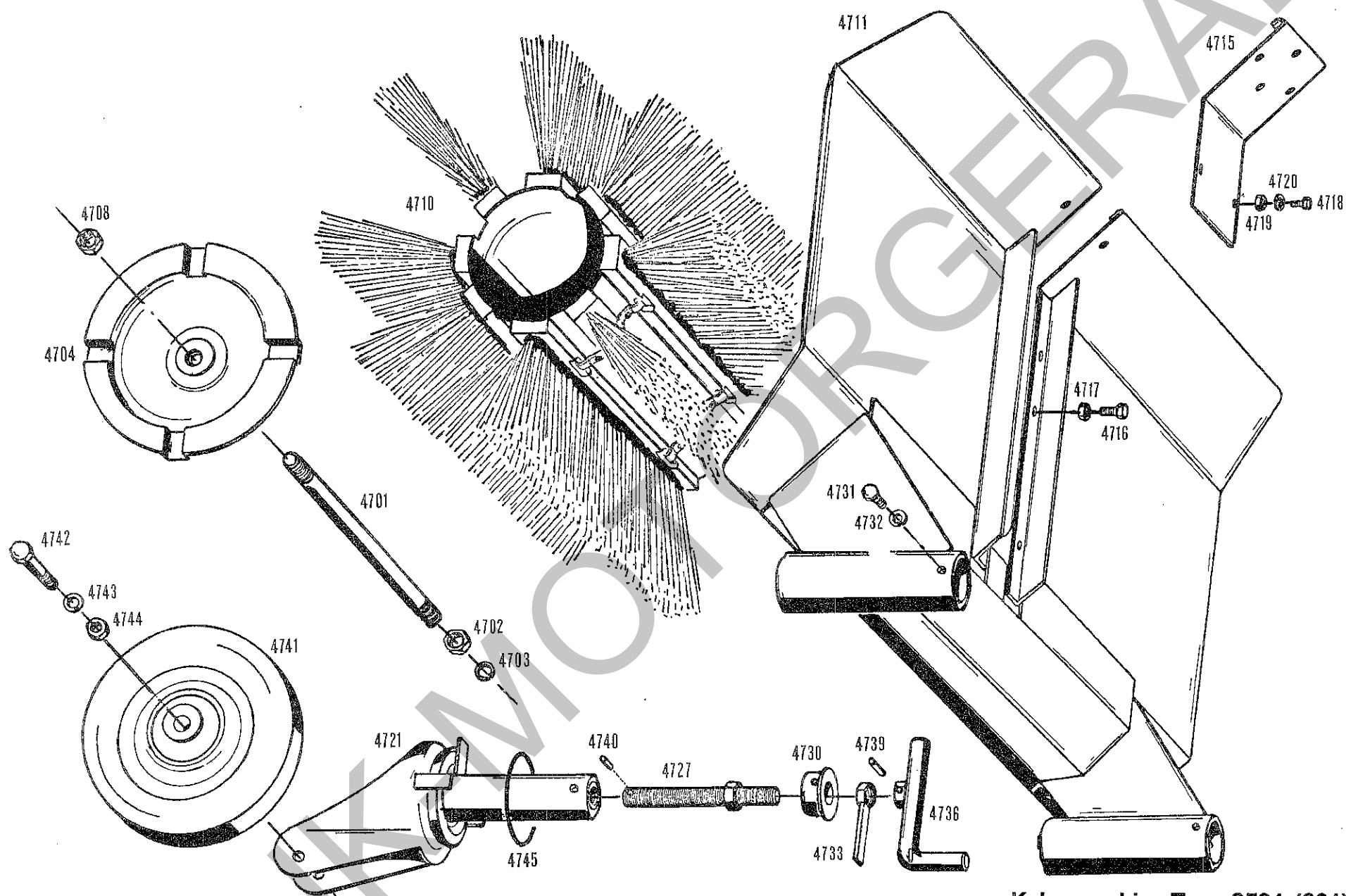
Kehrmaschine Type 3591 (801) Bildtafel No. 57
