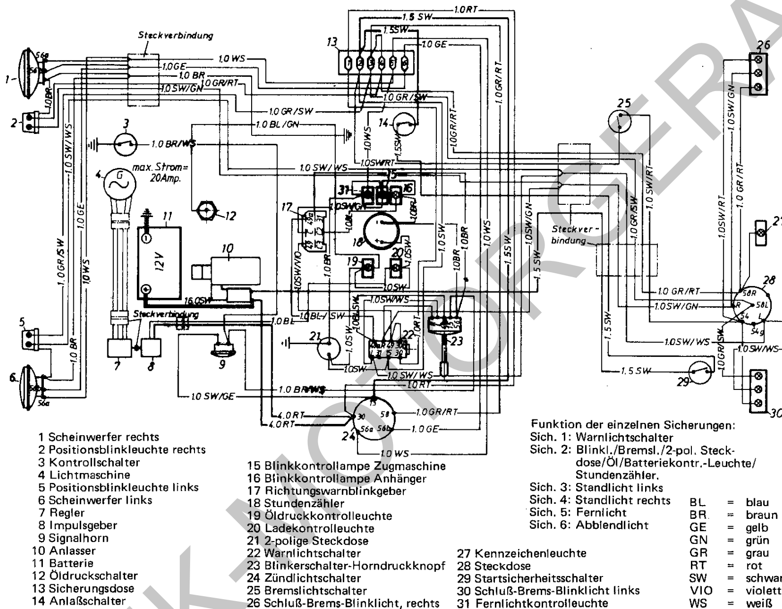
Schaltplan ab B 19 1222326 Bildtafel No. 27 a
