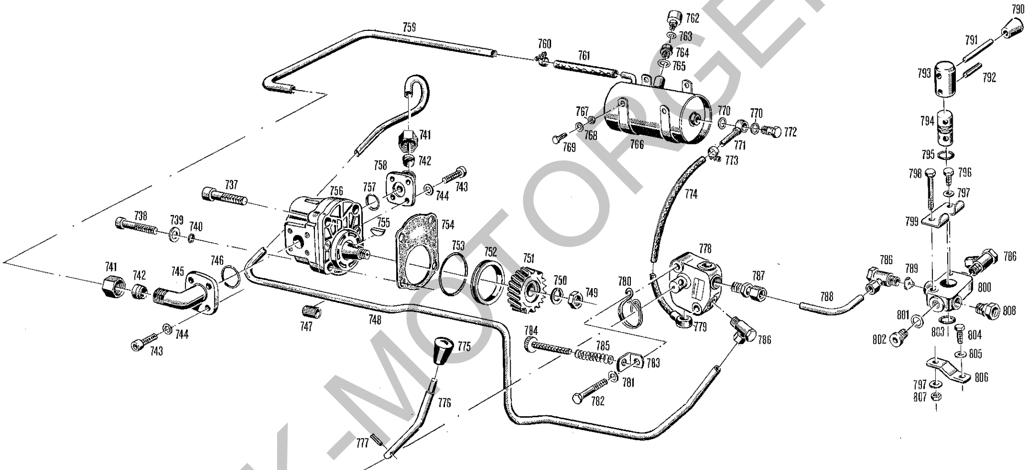
Bildtafel No. 11 Bis B 18-1222325
