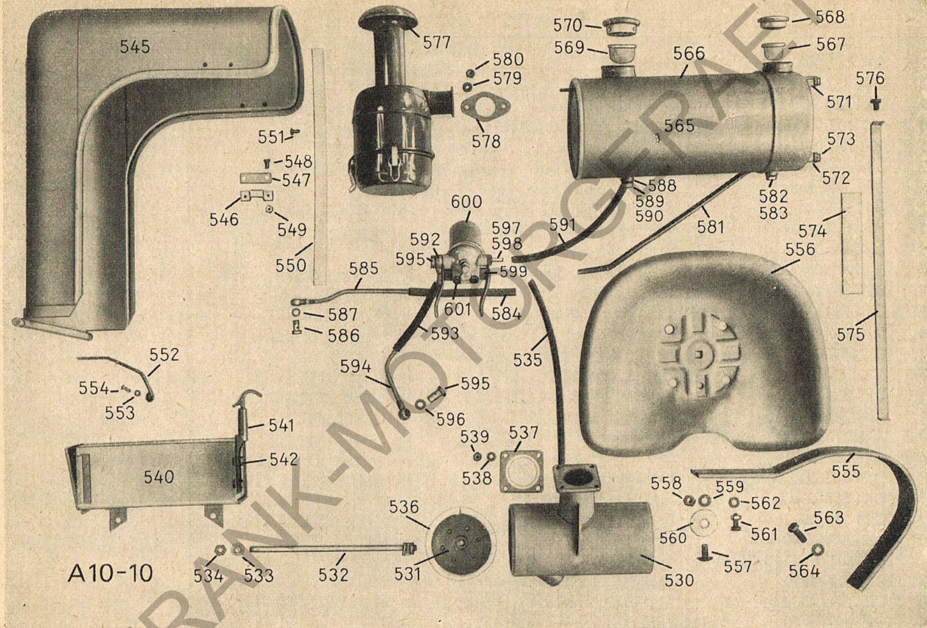
Tafel 7: Motorfortsetzung - Blechanbauten
