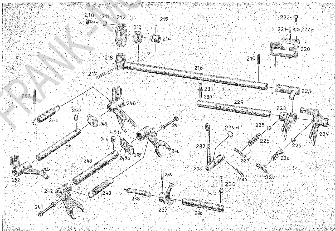
Tafel 4: Schaltung
