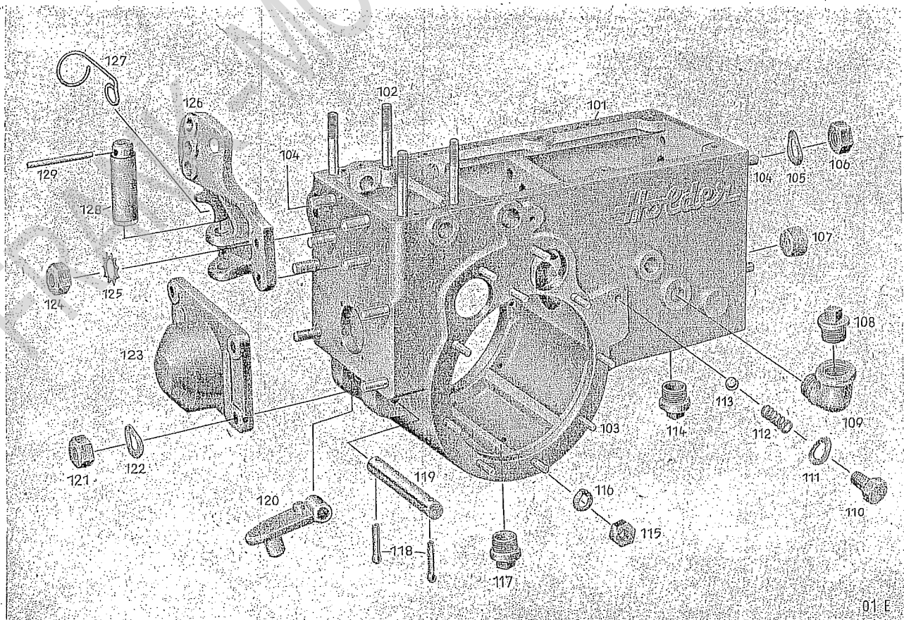
Tafel 1: Hauptkörper — Anhängervorrichtung — Flanschdeckel
