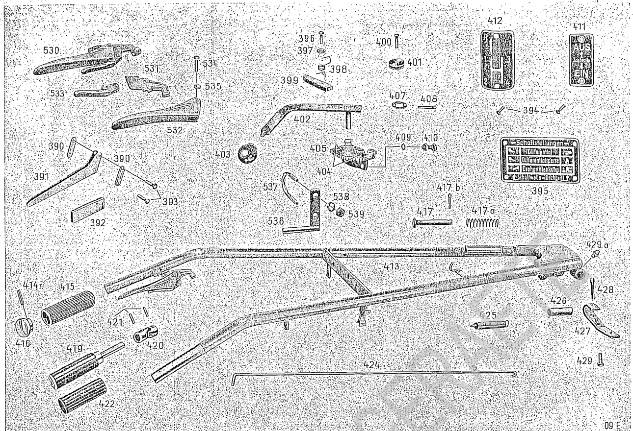
Tafel 9: Holme mit Bedienungsteilen
