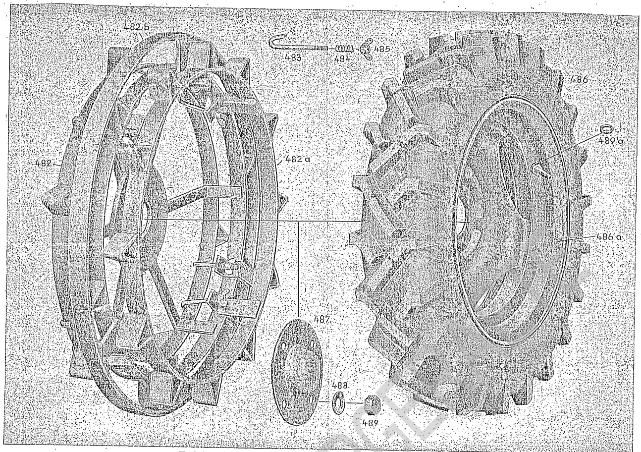
Tafel 13: Stahlgreiferräder und gummibereifte Räder
