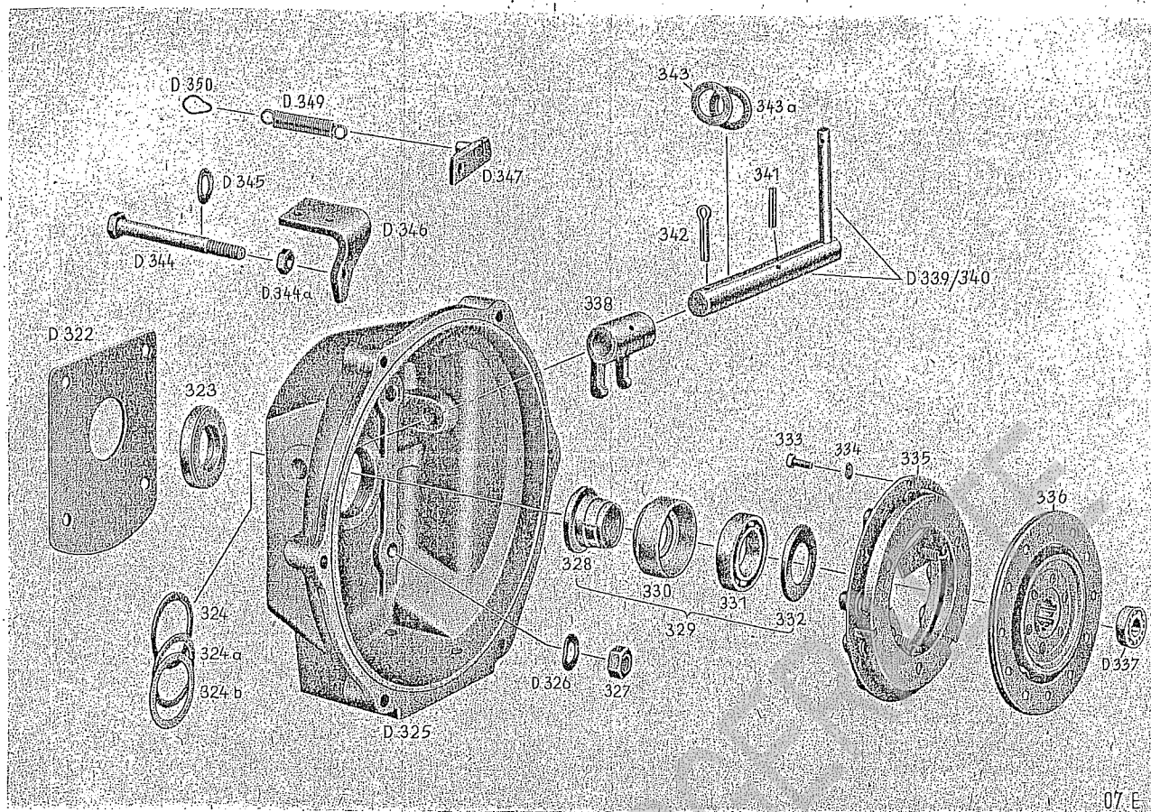
Tafel 7: Kupplungsgehäuse — Kupplung
