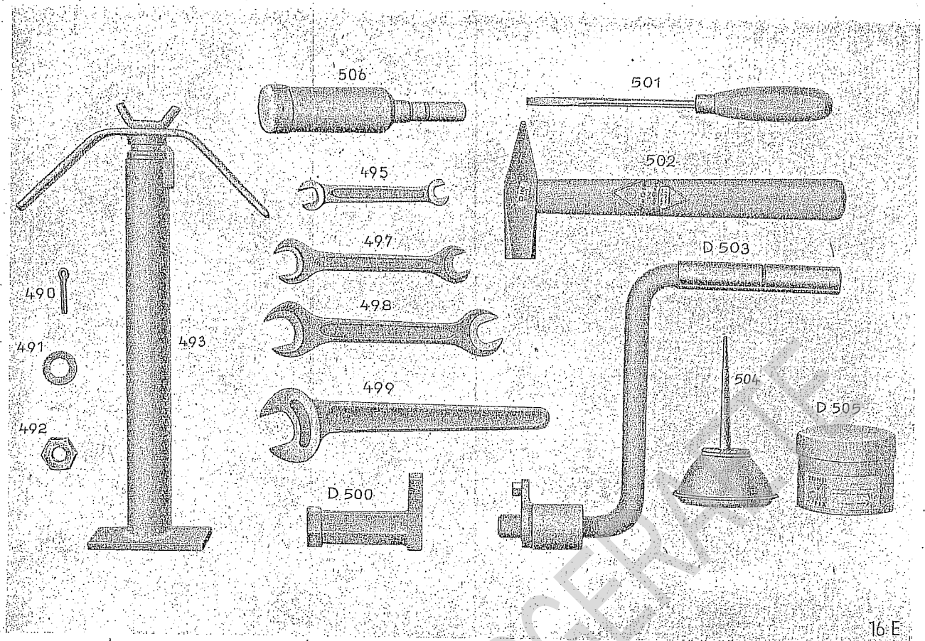
Tafel 16: Werkzeug und Zubehör
