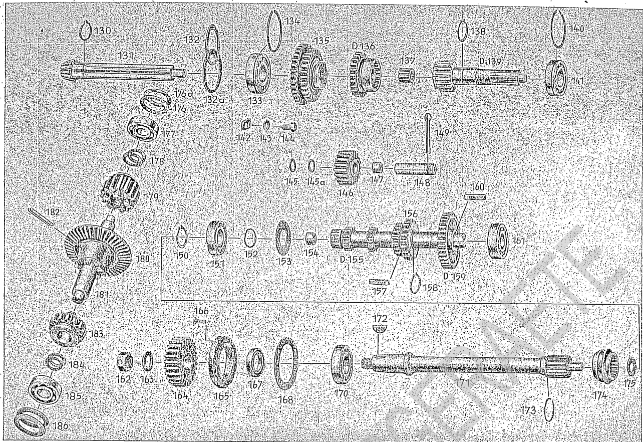
Tafel 2: Schalt- und Kegelradgetriebe — Zapfwelle
