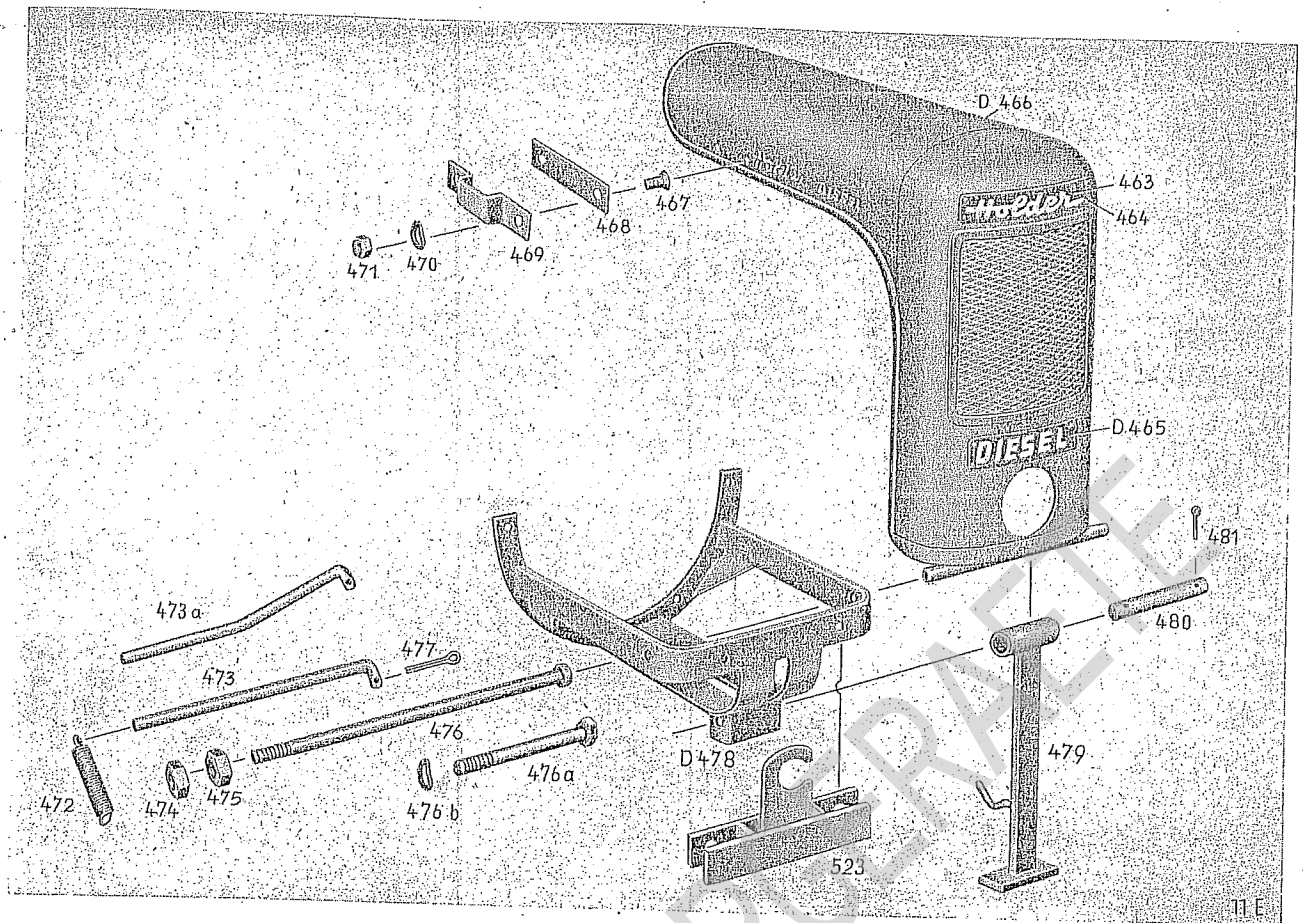
Tafel 11: Schutzbügel mit Stütze — Haube, alte Ausführung
