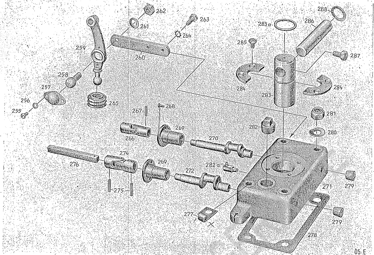
Tafel 5: Holmenlager
