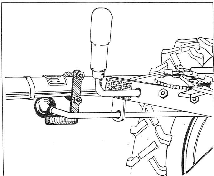
Sperre für Drehgriffenklung beim Einachsräumer BED II
